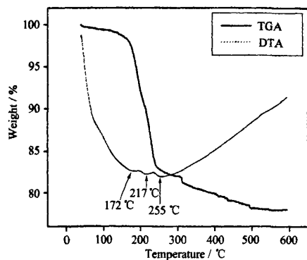
图 5 Cd(OH) 2 纳米棒的 TGA-DTA 图 Fig. TGA-DTA of Cd(OH) 2 nanorods
