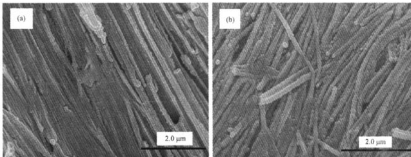
图 4 (a) 无电沉积 12 h 的 Cd(OH) 2 的 SEM 图, (b) 电沉积 1 h 的 Cd(OH) 2 的 SEM 图
